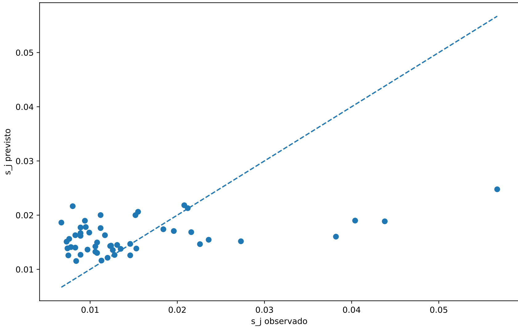
Shares observados vs previstos - logit simples
